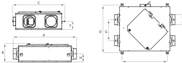
Bảng vẽ kỹ thuật
