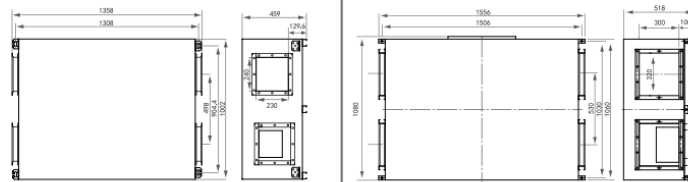
Bảng vẽ kỹ thuật
